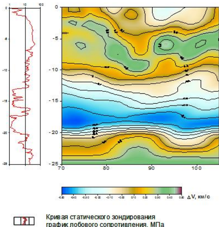
Рис.1. Сопоставление данных q_c и V_{ан}
