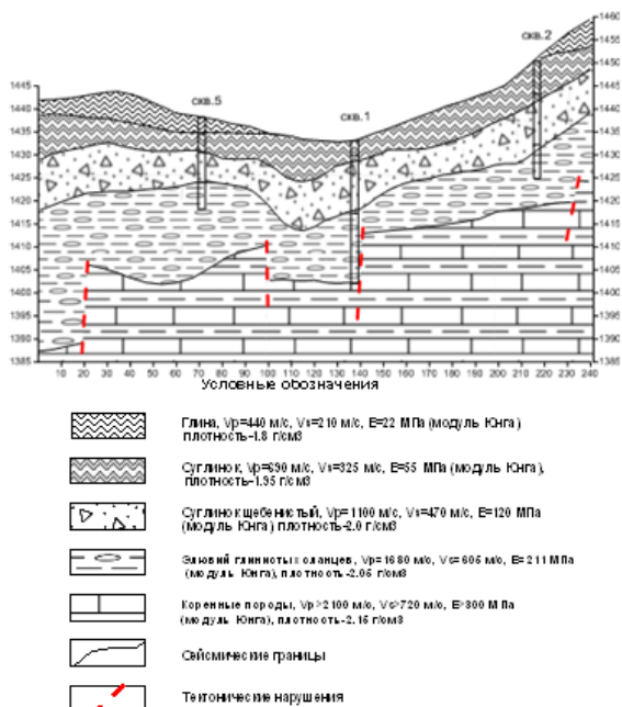
Рис. 8. Сейсмогеологический разрез по линии А-А
