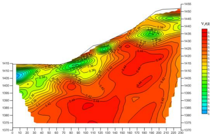
Рис. 9. Вертикальное сечение сейсмотомографической модели ( \nu )
