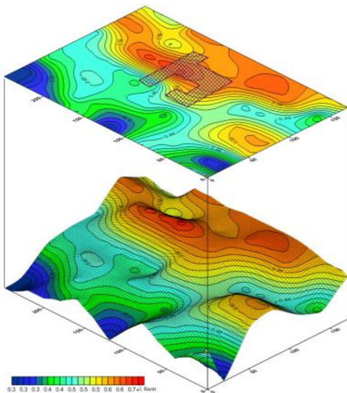
Рис. 12. Карта приращения сейсмичности
