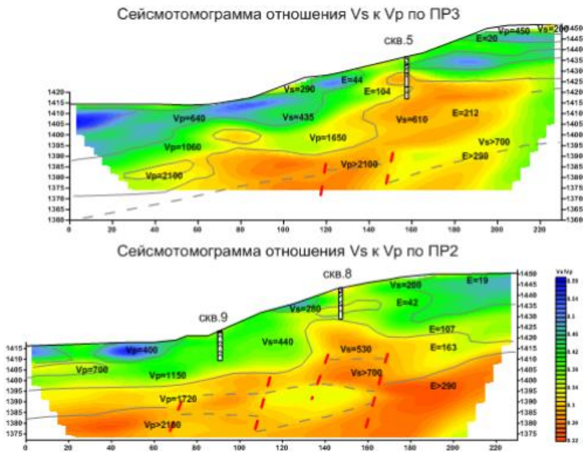
Рис. 6. Сейсмотомограммы \gamma = V_s/V_p
