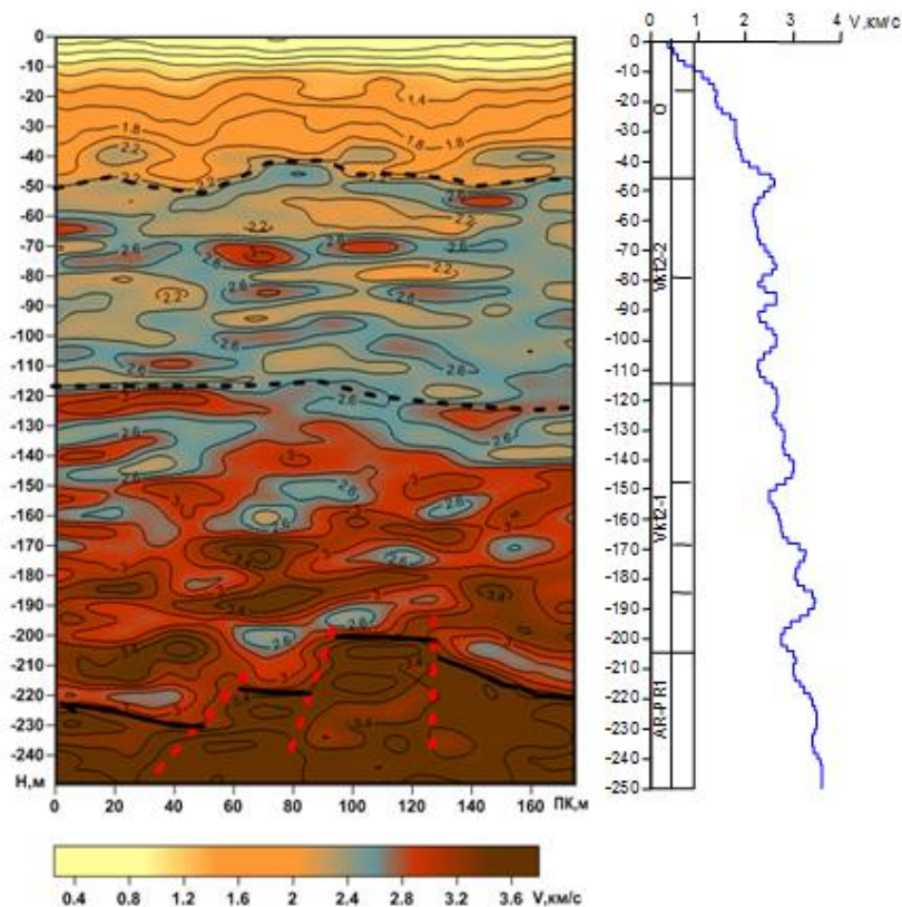
Рис.3. Особенности сейсмогеологического строения грунтов
