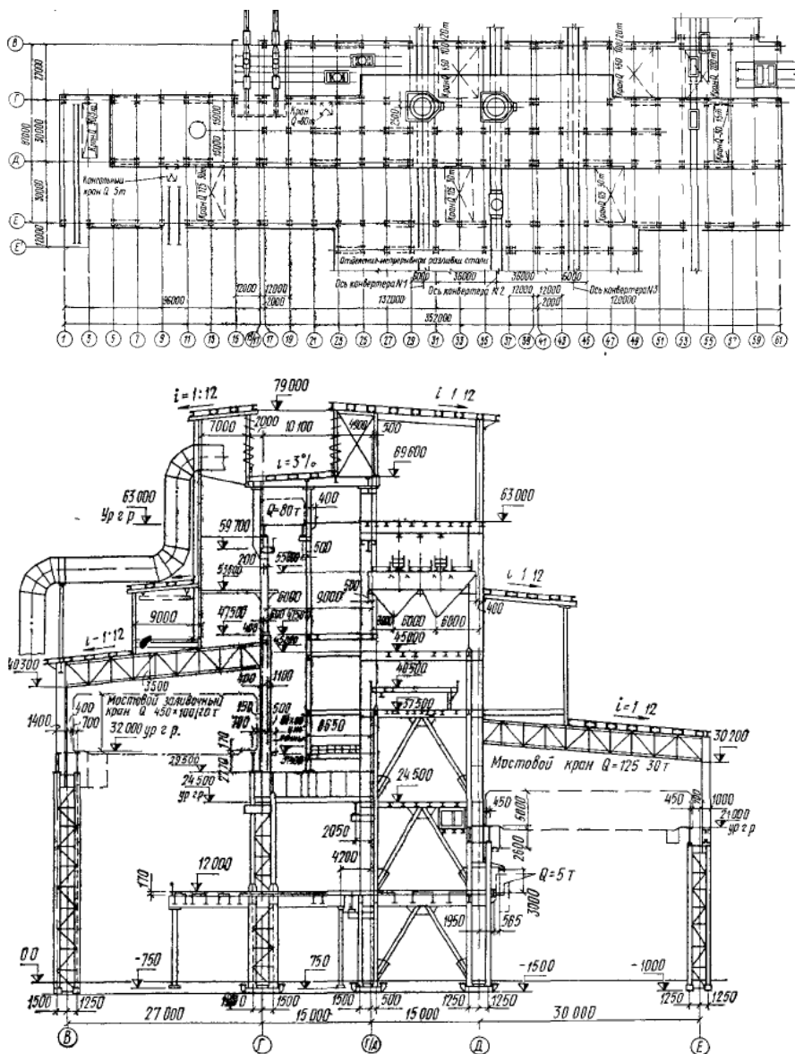
Рис. 2. План и поперечный разрез здания кислородно-конверторного цеха ОАО «ММК»
